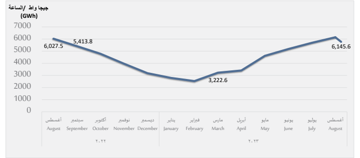
التغير في استخدام الكهرباء، أغسطس-٢٠٢٢ - أغسطس-٢٠٢٣ Change in Electricity Utilization, Aug. 2022 - Aug. 2023
